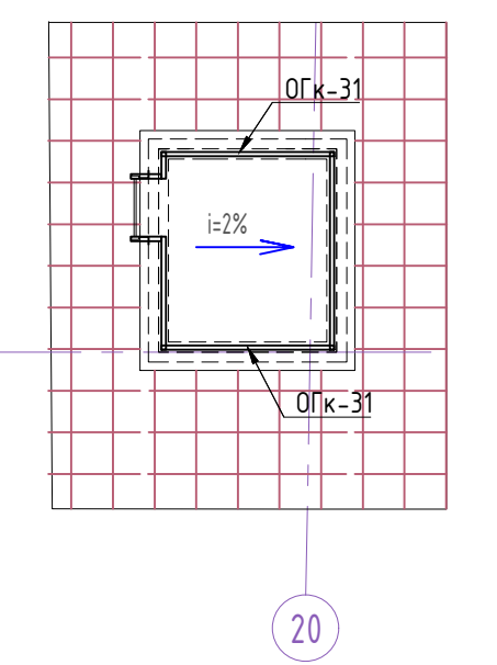
Паралет из железобетона
