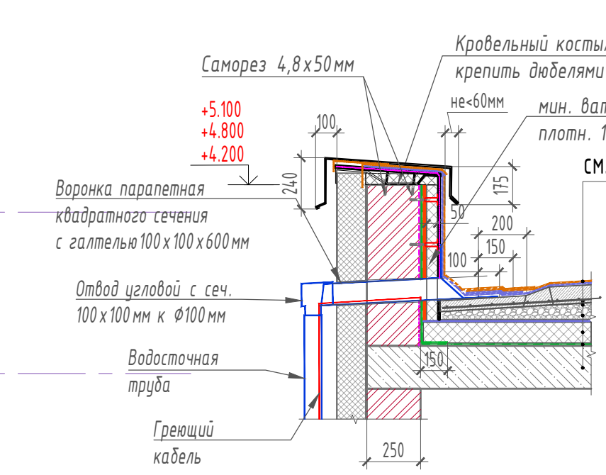
Устройство водоотведения через паралет кирпичный
