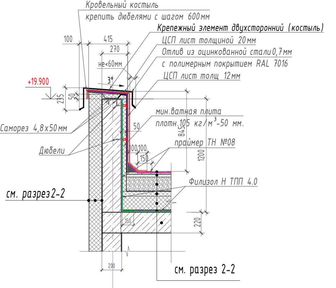
Паралет из железобетона
