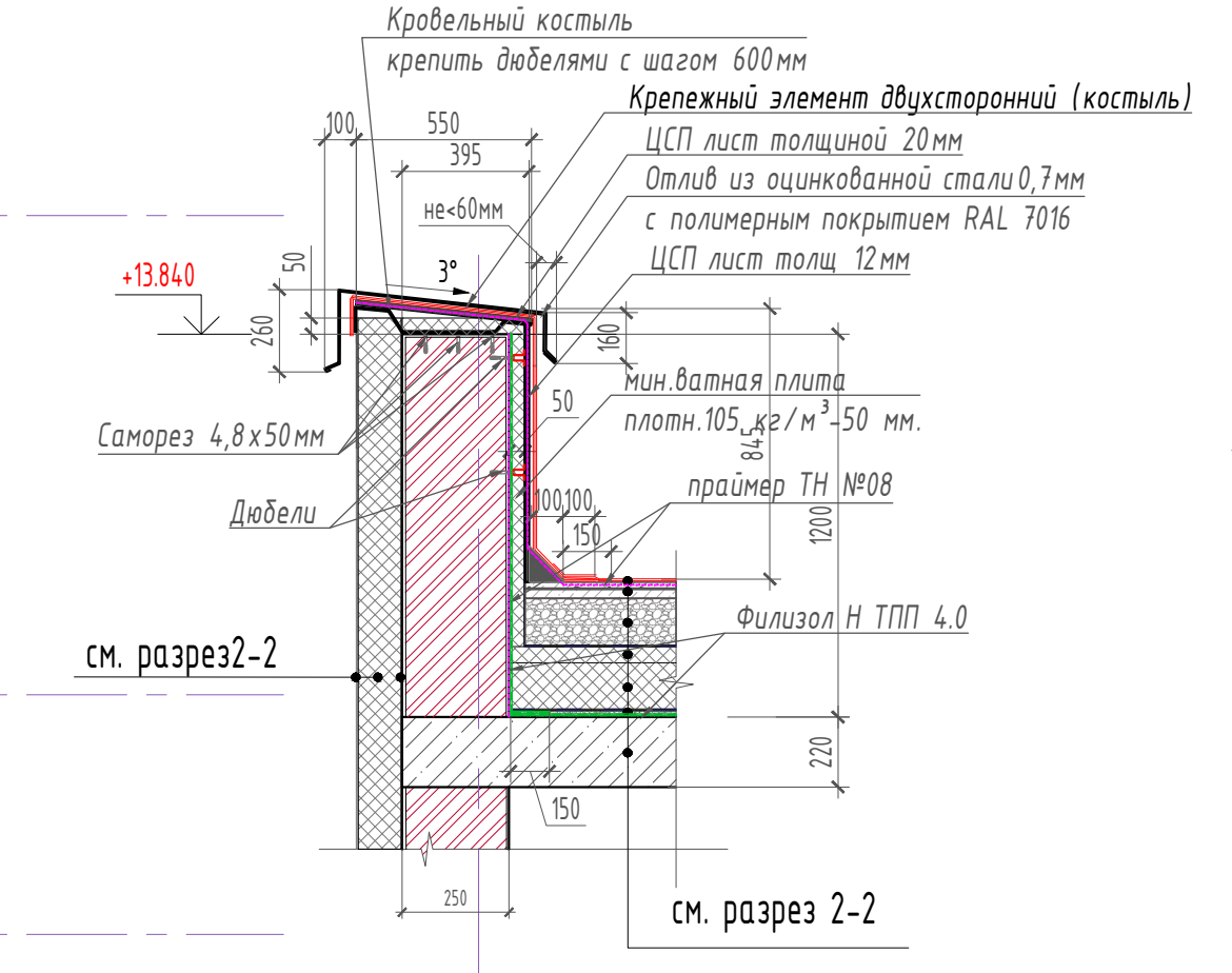
Паралет кирпичный
