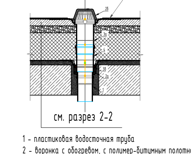
Узел 3
