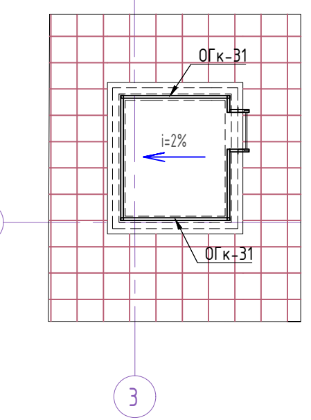
Фрагмент плана кровли в осях "З/Ж"
